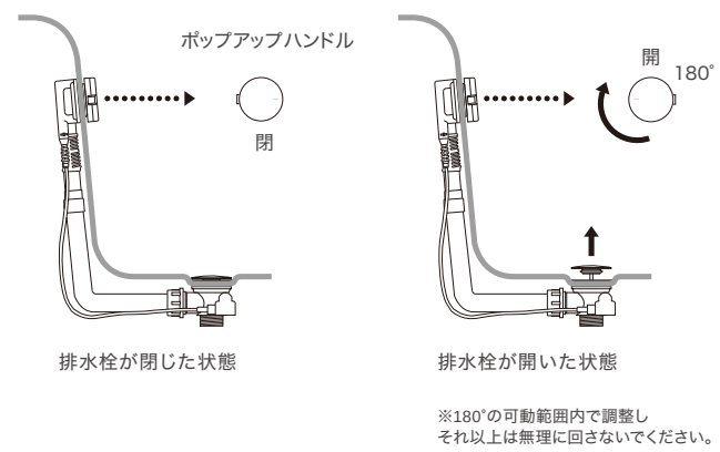
【ポップアップハンドルの操作について】
