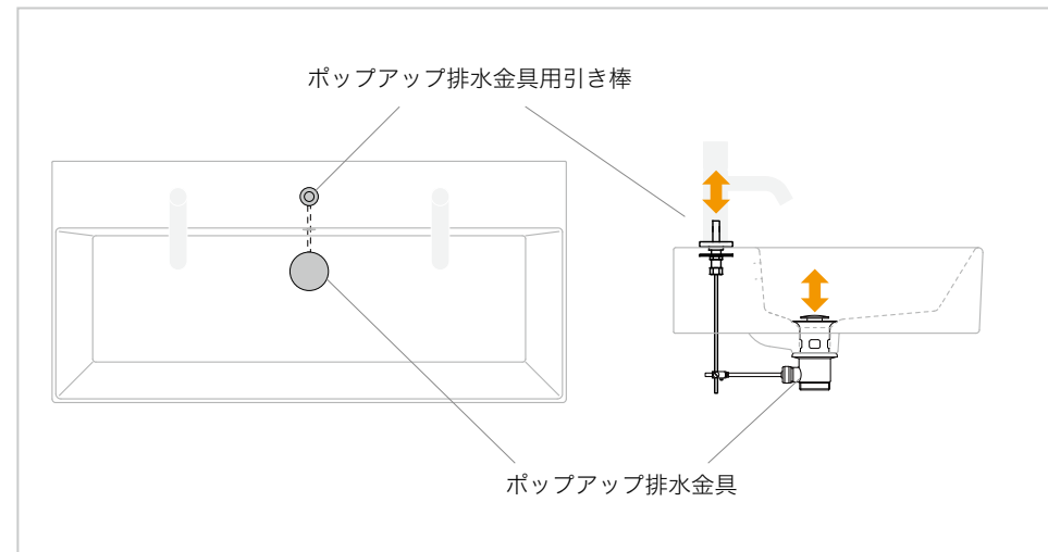
ポップアップ排水金具用引き棒 ARN73-9925 クローム ¥14,200
